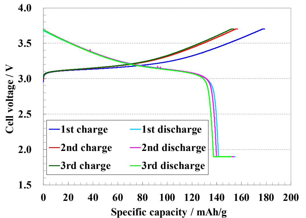
LiNbO 3 コート LiNi 1/3 Co 1/3 Mn 1/3 O 2 -Inハーフセル 0.1C CC-CV充放電試験@25℃
