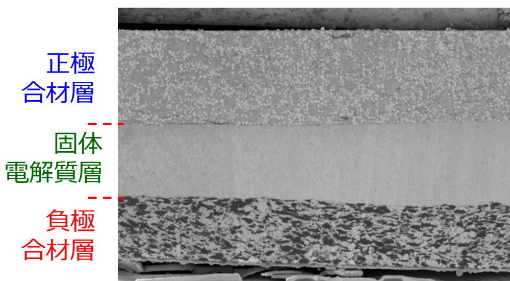
圧粉型全固体電池の断面SEM像
