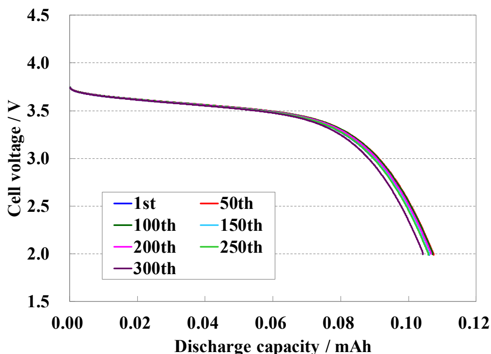
LiNbO 3 コート LiNi 1/3 Co 1/3 Mn 1/3 O 2 -グラファイトフルセル 充放電サイクル試験 1C×300サイクル@25℃
