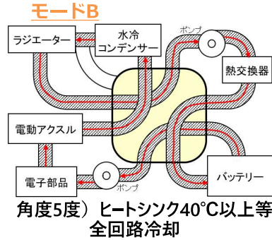
MBDモデル) バルブ角度 オクトバルブMBDモデルを搭載した車両熱マネシステムモデルの検証結果
