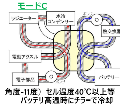
MBDモデル) バルブ角度 オクトバルブMBDモデルを搭載した車両熱マネシステムモデルの検証結果
